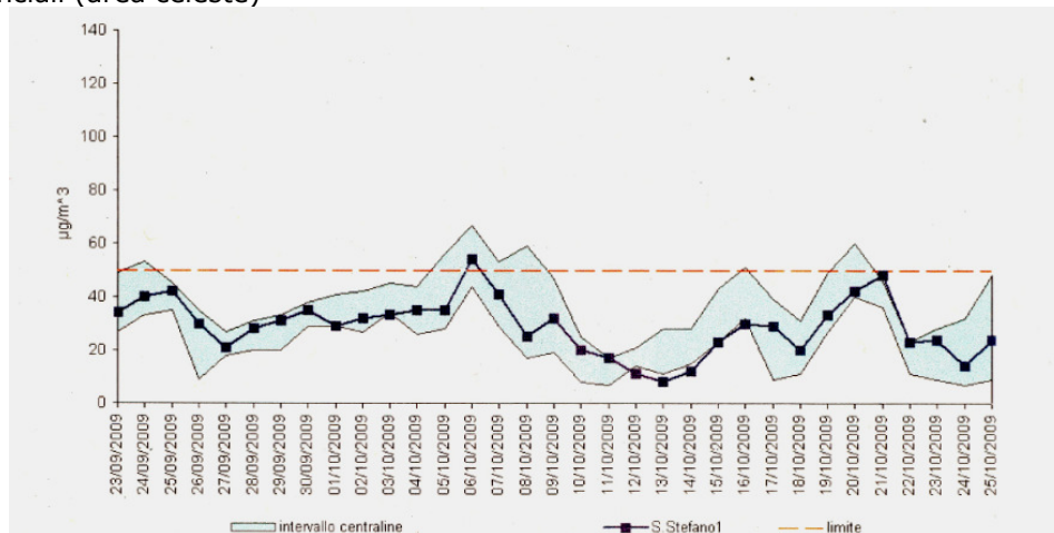
Fig. 18 – PM10: confronto tra concentrazioni medie giornaliere relative alla seconda fase (linea continua) e intervallo delle concentrazioni riscontrate nelle centraline fisse provinciali (area celeste)
