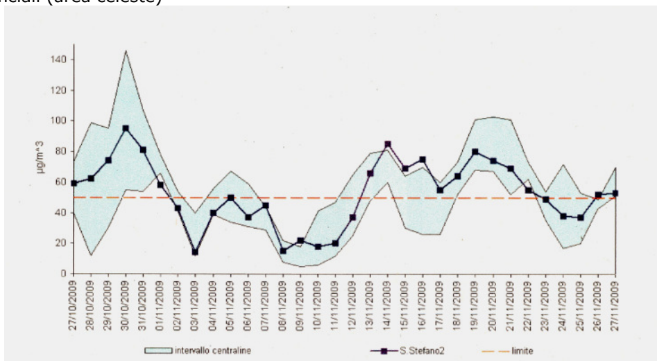
Fig. 18 – PM10: confronto tra concentrazioni medie giornaliere relative alla seconda fase (linea continua) e intervallo delle concentrazioni riscontrate nelle centraline fisse provinciali (area celeste)
