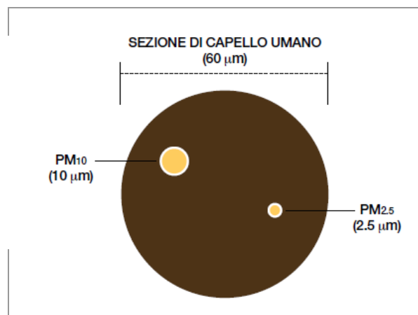
Fig. 1 - Confronto dimensionale tra la sezione di un capello umano e le due frazioni di particolato PM 10 e PM 2,5
